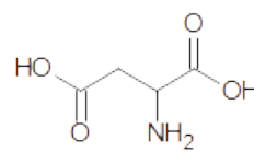
Asparaginsäure
