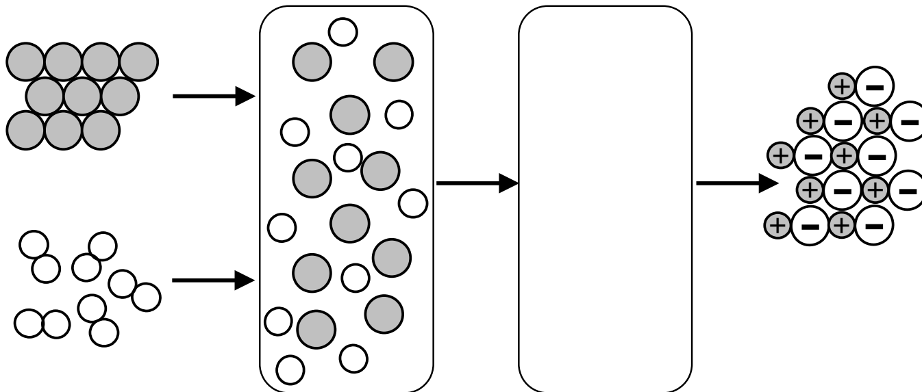
Abb. 2: Bildung von Natriumchlorid aus den Elementen, gedanklich zerlegt in Einzelschritte. Quelle: Eigenes Werk
