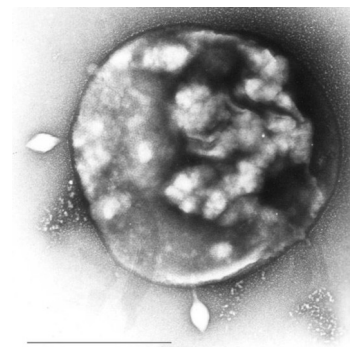
Abb. 2: Ein Archaeon wird von Viren infiziert Q: wikicommons, A:Xianguyux
