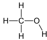
b) Methanol
