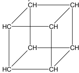
e) Cuban
