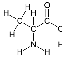
g) Alanin
