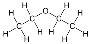
f) Diethylether
