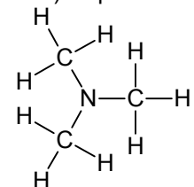
l) Trimethylamin
