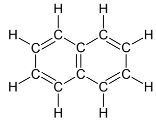
h) Naphtalin
