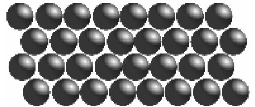
Abb. 1: Teilchenmodell eines Feststoffs: Kristall
