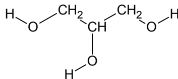
j) Glycerin
