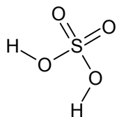
i) Schwefelsäure
